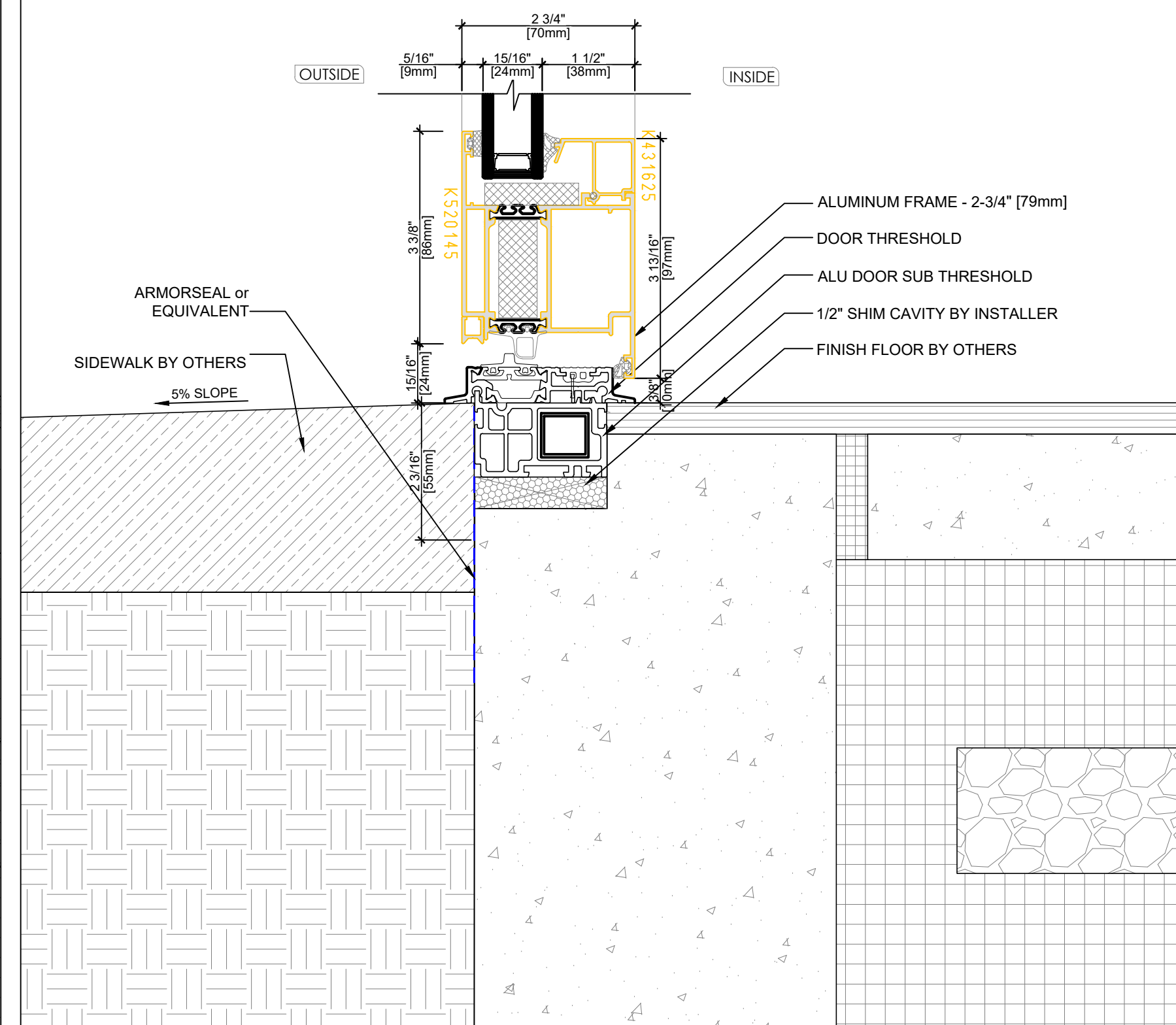
2B Option B: ENTRY DOOR SILL DETAIL DG-ALU79-1 SCALE: 1:2
