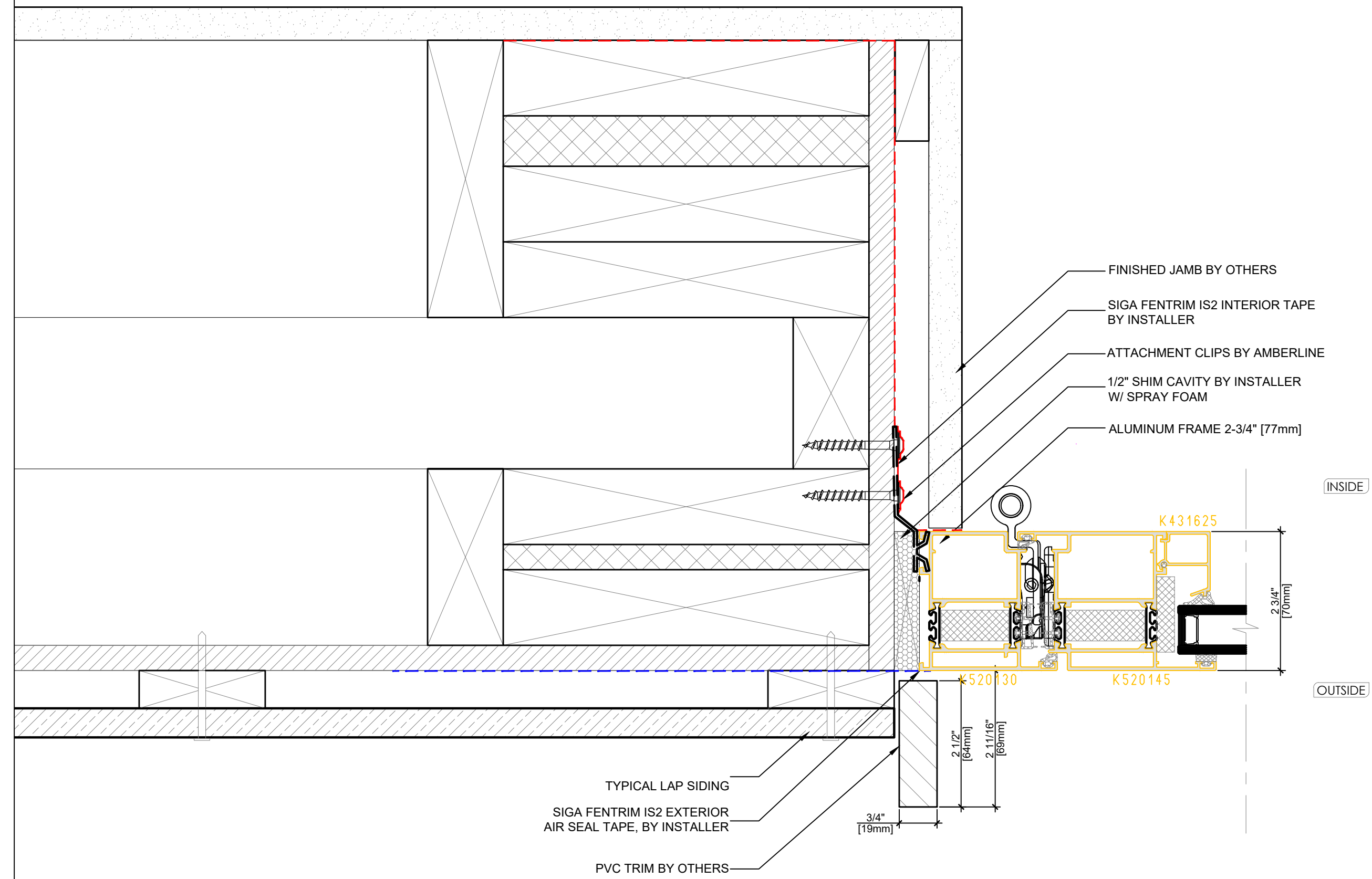
3 ENTRY DOOR JAMB DETAIL DG-ALU79-1 SCALE: 1:2
